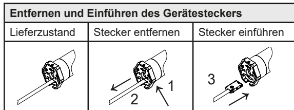
Fig. 4 Entfernen und Einführen des Gerätesteckers
