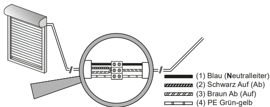
Fig. 7 Anschluss Funksendebetrieb
