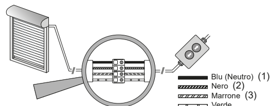
Fig. 6 Allacciamento per cavi di montaggio
