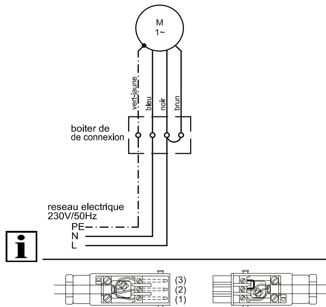
Fig. 5 Schéma des connexions RolMotion/D+ M-868 230 V / 50 Hz et disposition du câble lors de l'utilisation d'un connecteur Hirschmann STAS-3 (vec pontage)
