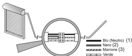
Fig. 7 Collegamento radio (modalità trasmettitore)
