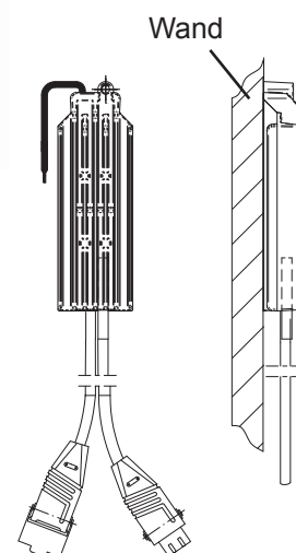
Empfohlene Einbaulage
